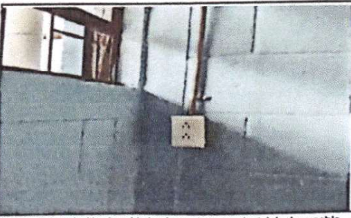
FOTO 10: Instalación de unidades fuerza (tomacorriente). Incluye cable eléctrico en aula
